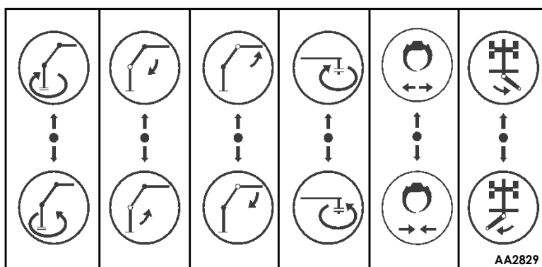
Figur 3:3 Flerspåk (6 sektioner)
