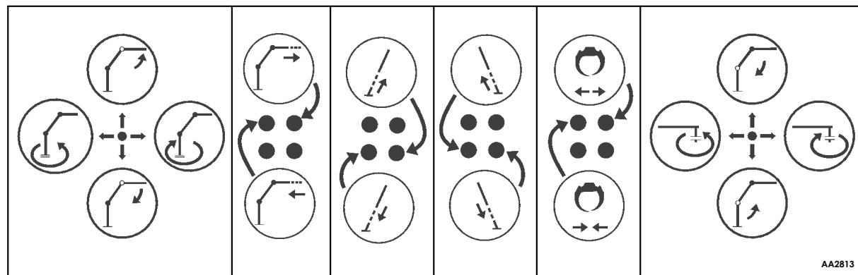
Figur 3:6 Lågtrycksservo (PCL)
